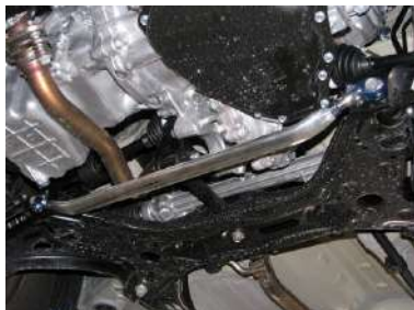
[ロアアームバー フロント] KAWAI WORKS製品。 左右ロアアームを繋ぎます。
