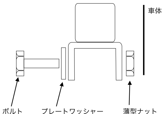
延長ブラケット
