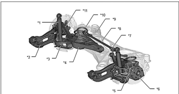
リア (FF車)
