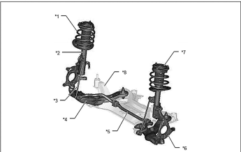
フロント
