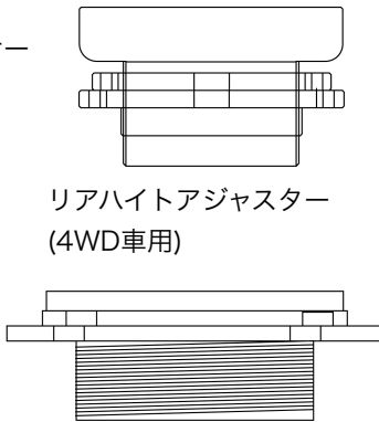
リアハイトアジャスター (FF車用)
