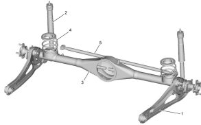
リア(4WD車)
