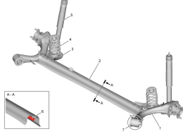
リア(4WD車)
