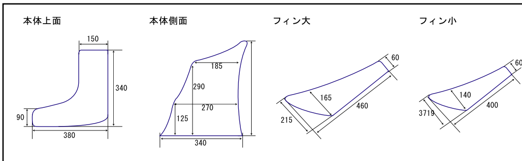
汎用フロントカナード 構成部品&寸法図
