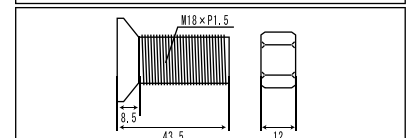
寸法図(アダプター type-2)
