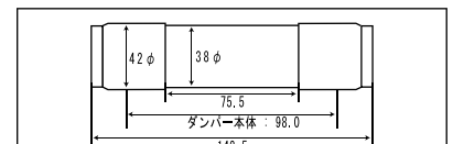
寸法図(ダンパー本体)
