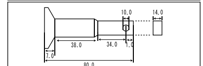
寸法図(アダプター type-1)
